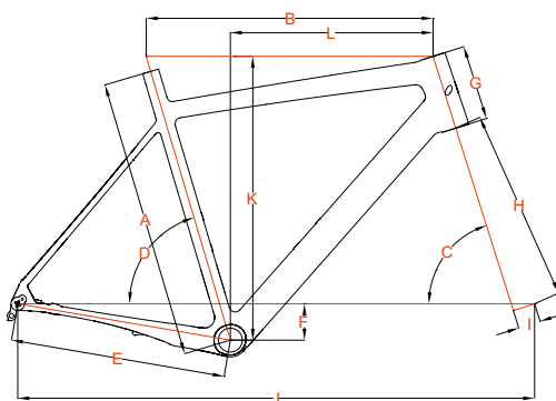
Размеры велосипеда Fitness Bike Crater Lake / Trekking Bike Aventura
